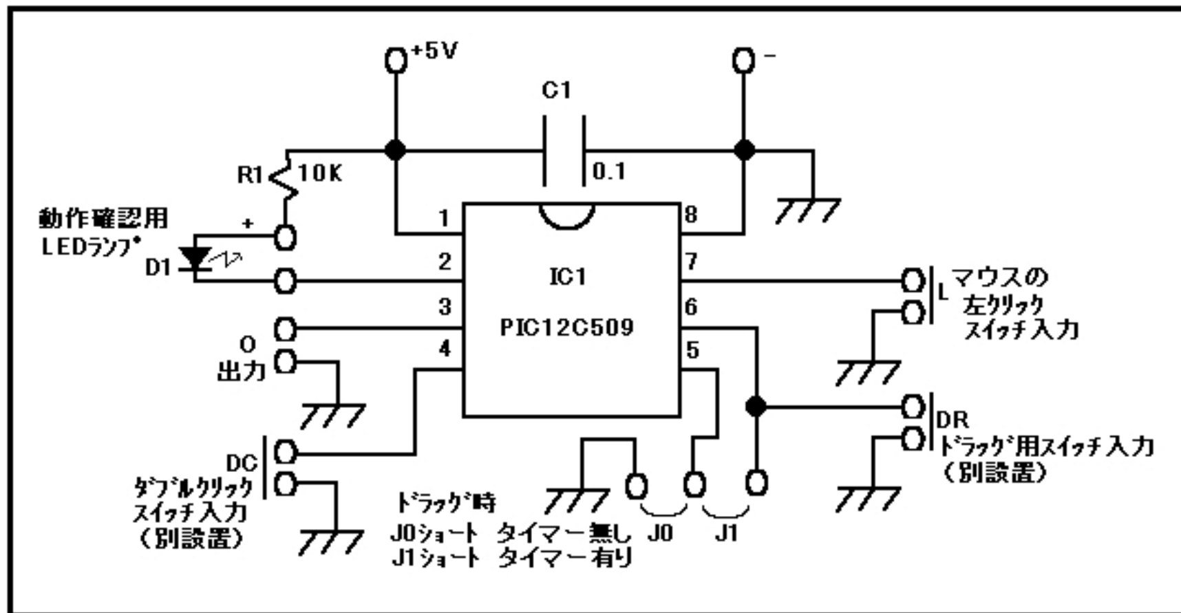
CCC回路図
