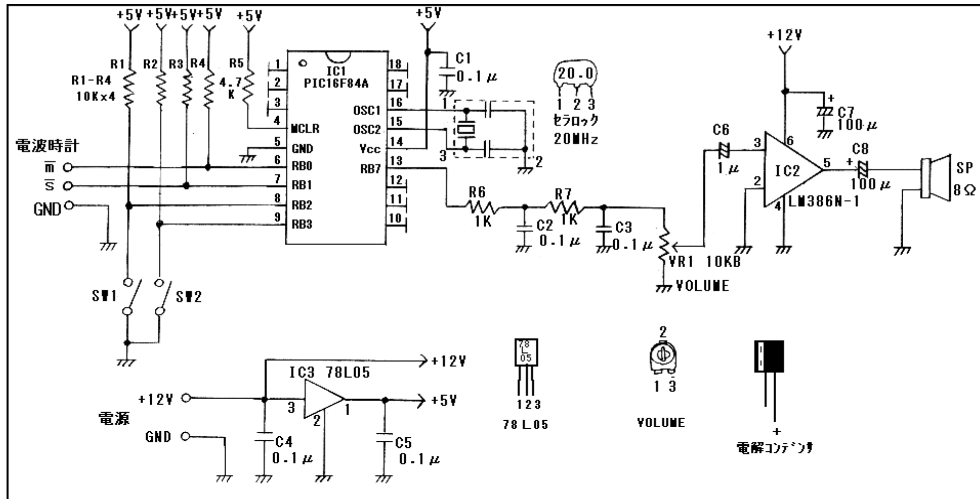
JJY もどき音響器回路図
