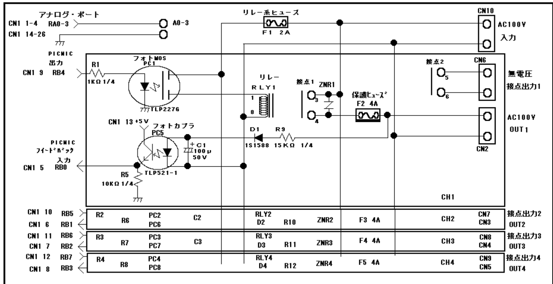
ACテーブル・タップ回路図
